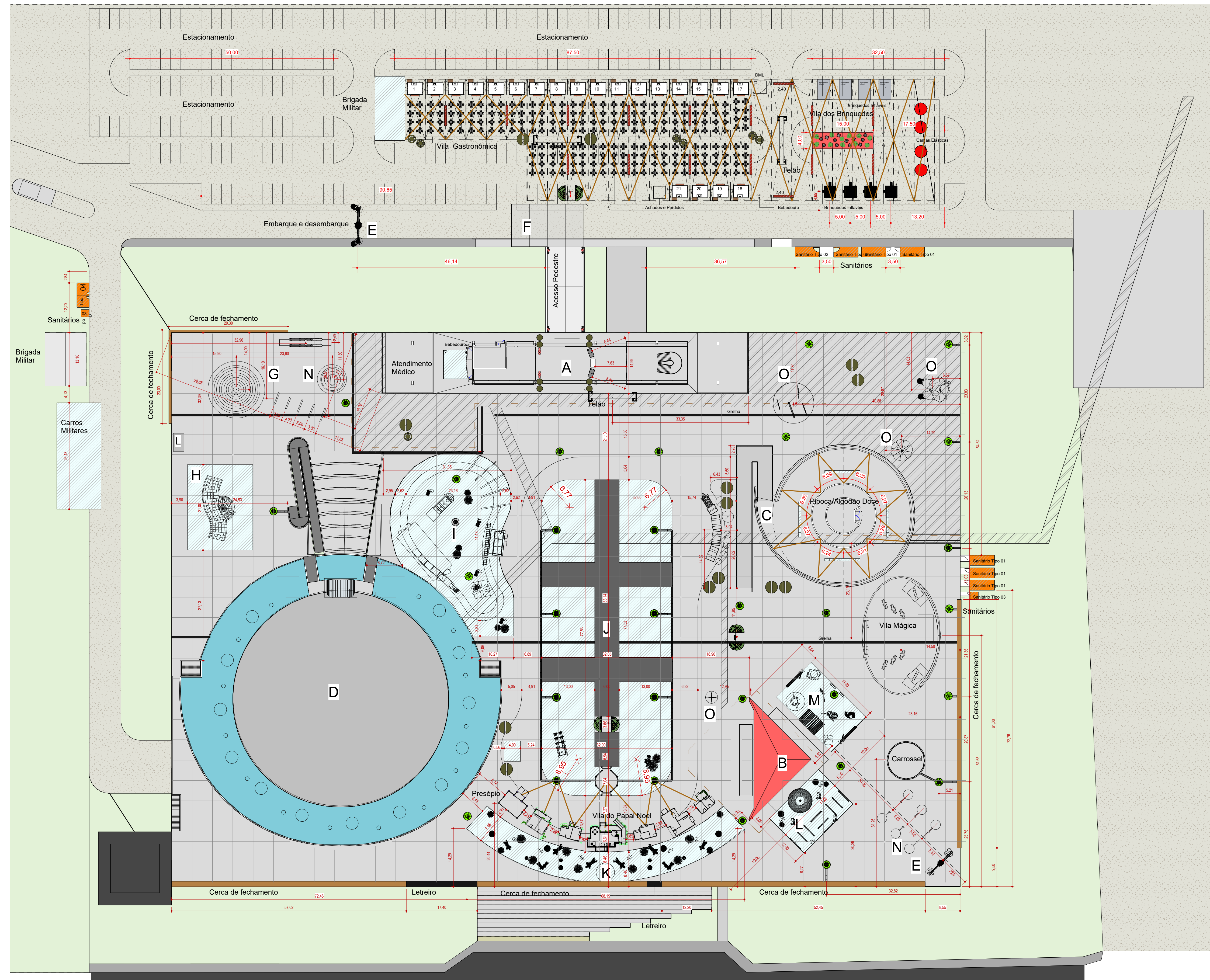
1 PLANTA DE LOCAÇÃO DE EQUIPAMENTOS - COTAS 1 : 500
