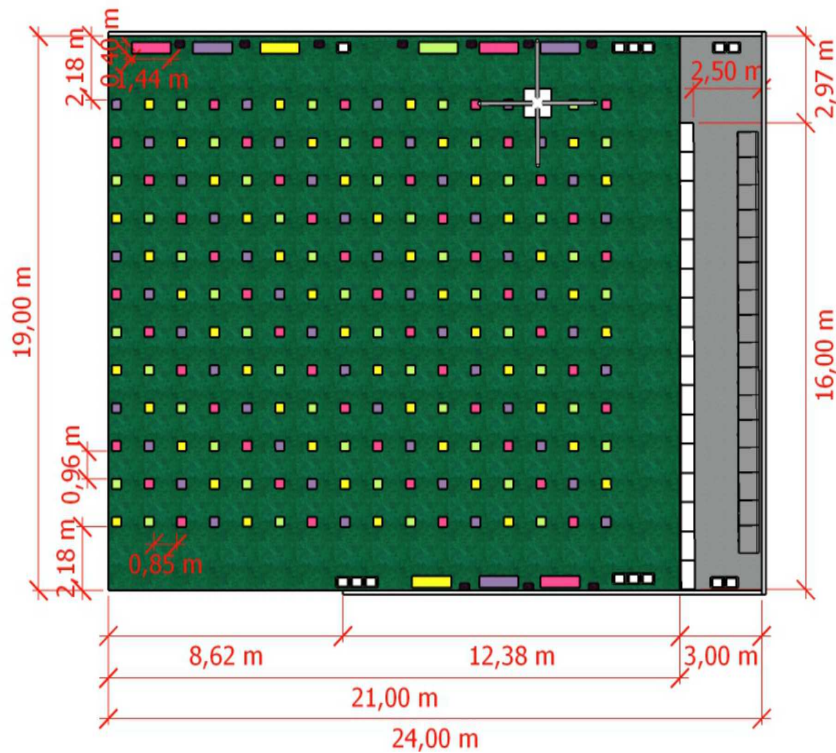
VISTA SUPERIOR
