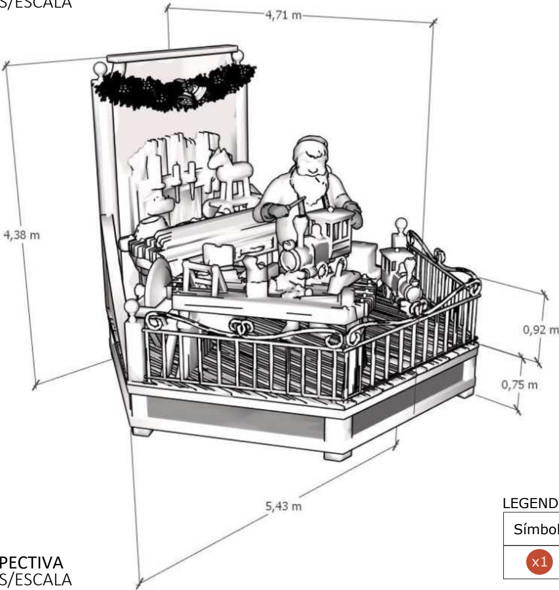
PERSPECTIVA Esc.: S/ESCALA
