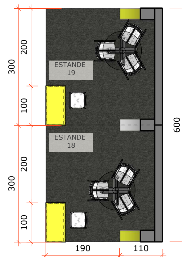
Estandes Amarelos - Planta Baixa Esc.:1/60
