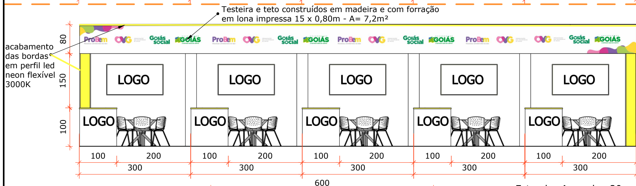
Estandes Amarelos:20 ao 24 Vista Frontal Esc.:1/60
