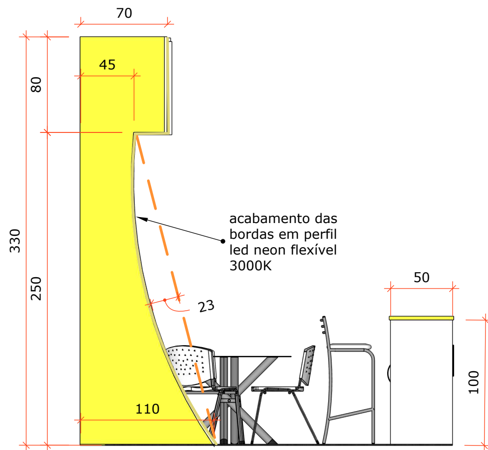
Estandes Amarelos - Vista Lateral (052) Esc.: 1/30
