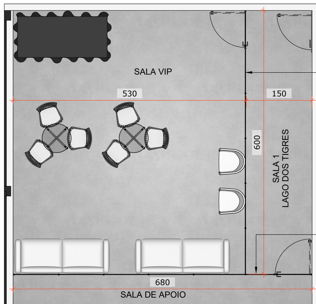
Sala Vip Planta de Layout Esc.:1/50 0157
