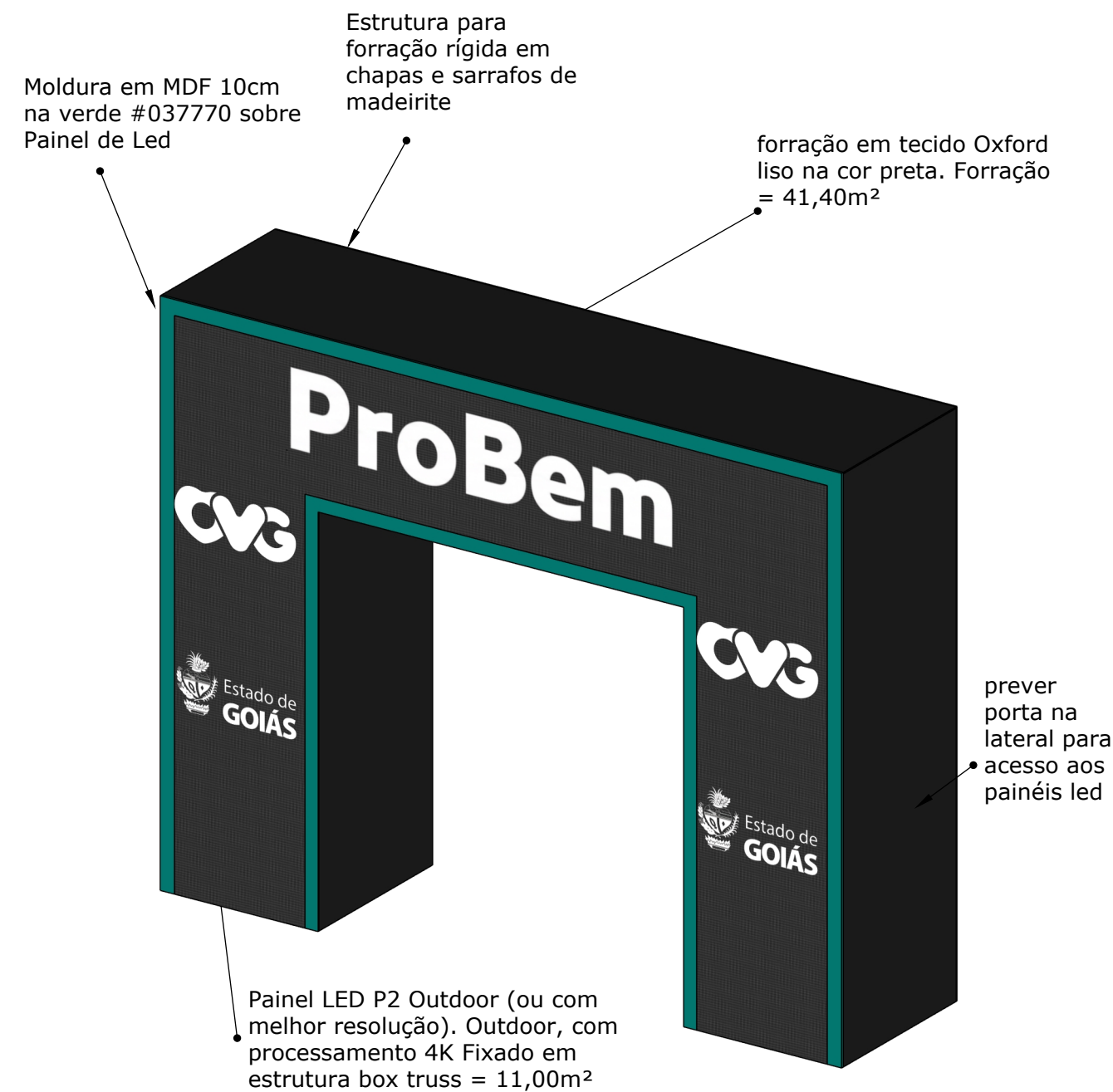
02 Persp. Frontal - Forração Pórtico Entrada Sem Escala
