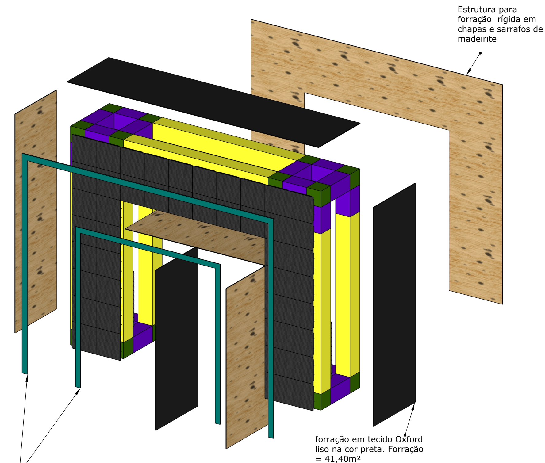
06 Persp. Frontal - Forração/Estrutura Pórtico Entrada Sem Escala
