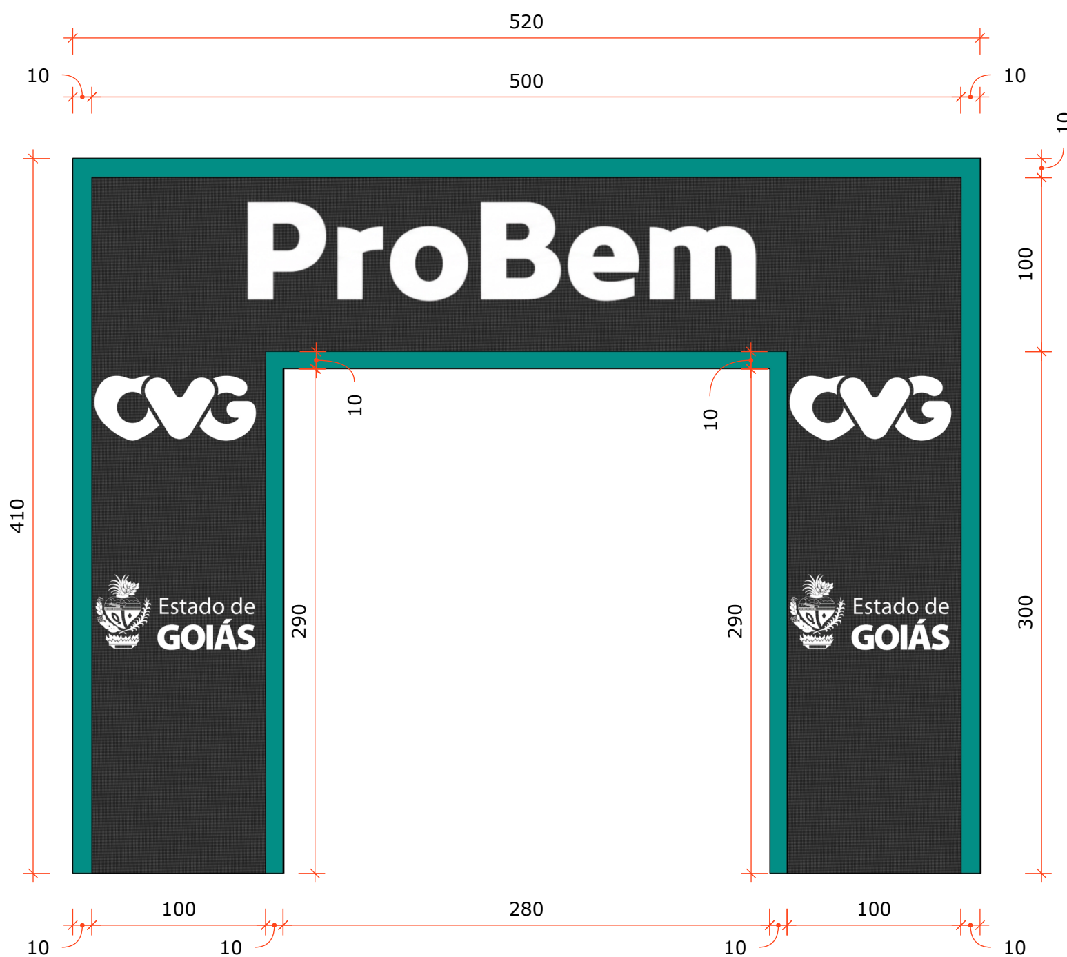
01 Vista Frontal - Forração Pórtico Entrada Esc.: 1/30
